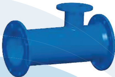
Formstück mit angeschweißtem Flanschabgang* (z.B. FF, T, TT, Reinigungskasten) Fitting with welded flanged branch* (eg. FF, T, TT, hatch box)
