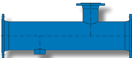
z.B.: FF-Stück mit Nabe und seitlichem Flanschabgang (max. 2000 mm) e.g.: FF double-flanged pipe with boss and side flange outlet (max 2000 mm)
